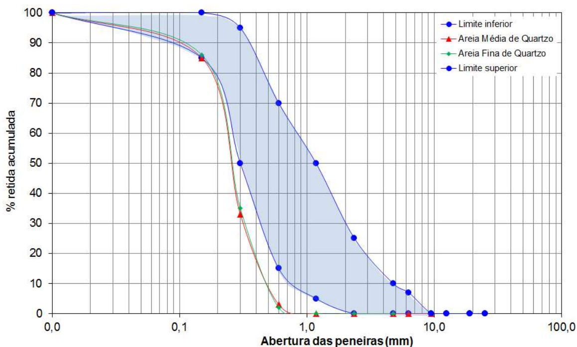
FIGURA – Ilustração das curvas granulométricas
